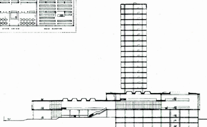
попечни пресек
